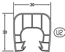
Connecteur U polycarbonate NG
