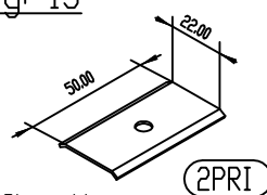
Plaque de répartition
