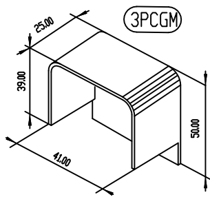
Bouchon pour connecteur Polycarbonate (3PCGM)
