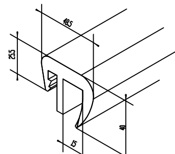
Joint Néoprène pour Tympan
