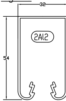
Connecteur U aluminium pour DP8, DP10 et DP16
