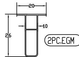
Ecarteur polycarbonate pour connecteur U polycarbonate grand modèle
