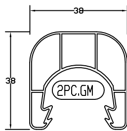
Connecteur U polycarbonate grand modèle
