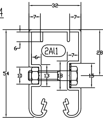
Connecteur U aluminium pour DP8, DP10 et DP16
