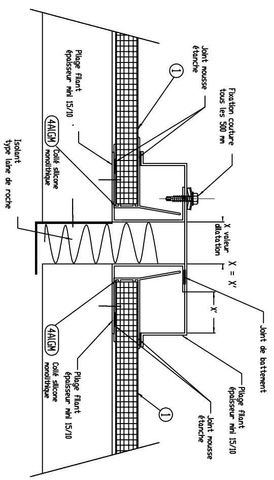
Coupe horizontale (panneau tronqué)
